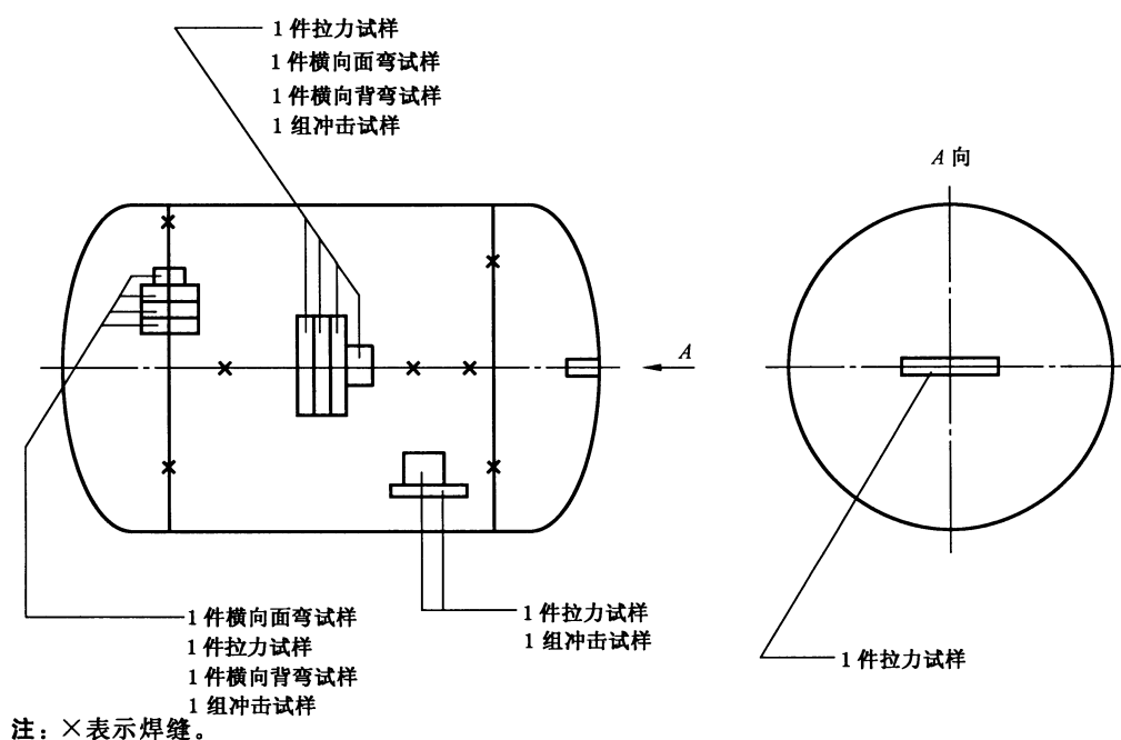
图 11 有纵焊缝钢瓶的取样位置示意图
